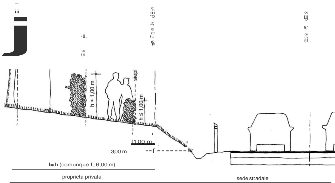
Distanze minime di impianto lungo il confine stradale al di fuori dei centri abitati
