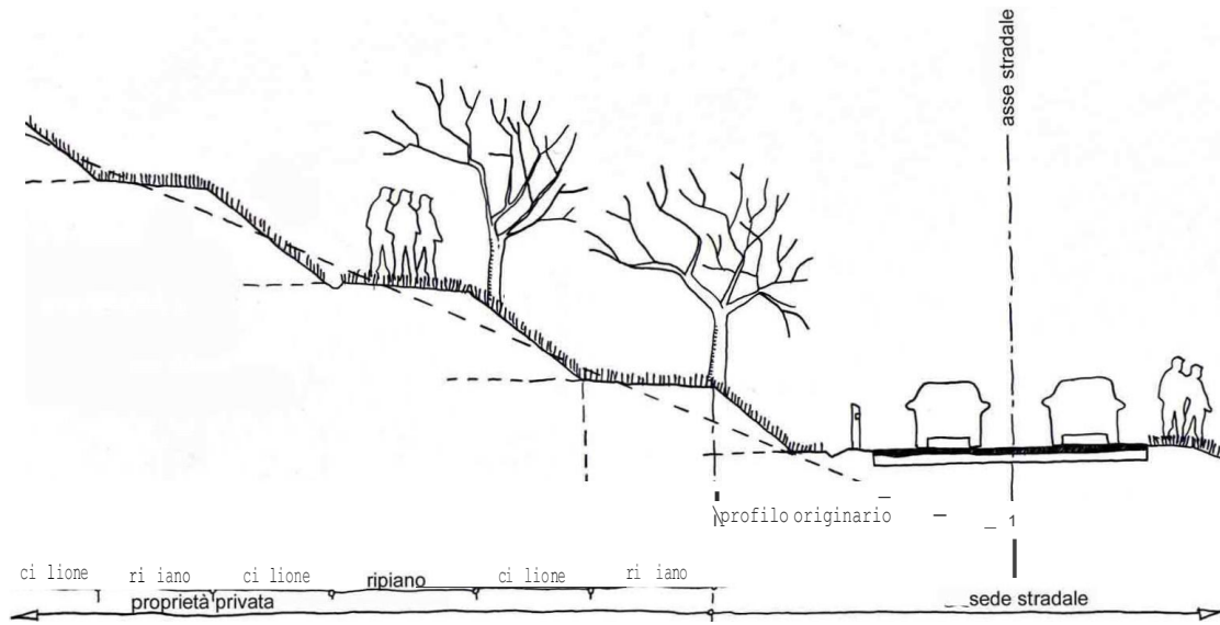
Sistemazioni in pendio - Cigliani
