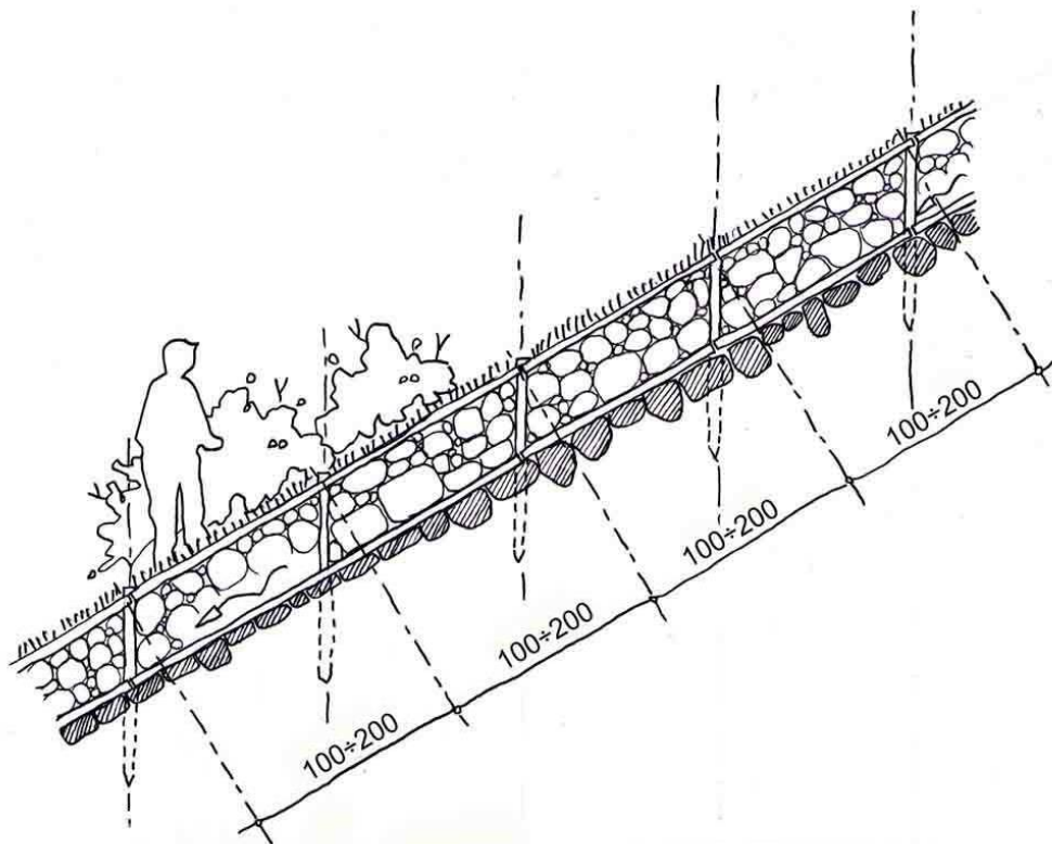
□ Profilo longitudinale
