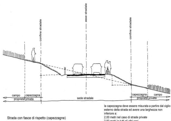
Strada con fasce di rispetto (capezzagne)
